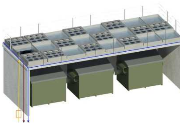
Abb. 1: Carport-Dachbegrünung - Wasserbecken mit installierten HPL® Pflanzmodulen
