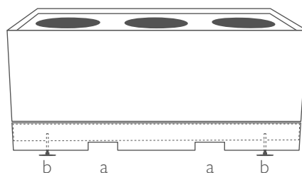
Unterkonstruktion mit Aussparungen (a) zum Transport mit einem Hubwagen oder Gabelstapler und zusätzlichen höhenverstellbaren Standfüßen (b) zur Niveauregulierung
