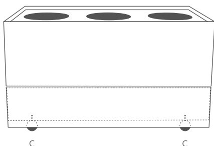
Unterkonstruktion mit verdeckten Schwerlastrollen (c)
