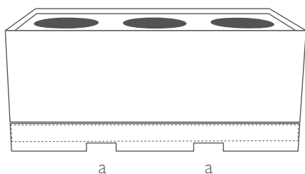
Unterkonstruktion mit Aussparungen (a) zum Transport mit einem Hubwagen oder Gabelstapler
